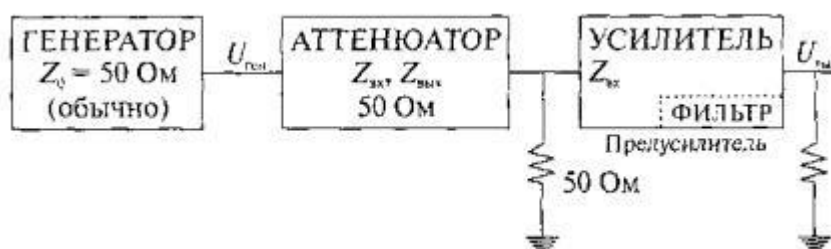
Рис. 1. Функциональная схема измерения параметров аппаратуры акустической эмиссии
